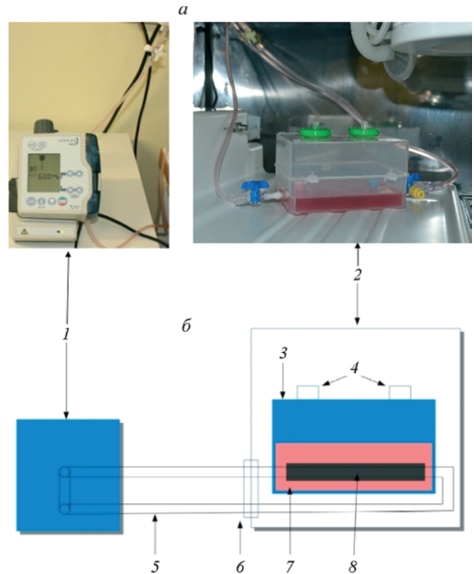
Рис. 1. Фотография (а) и схема (б) сконструированного биореактора.
